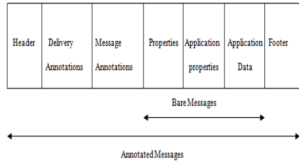
Fig.8. AMQP Message Format [1]
